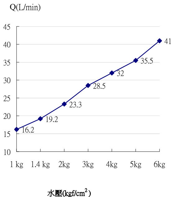
流量表
